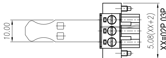
02~03P尺寸图
