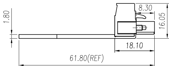
08~24P尺寸图
