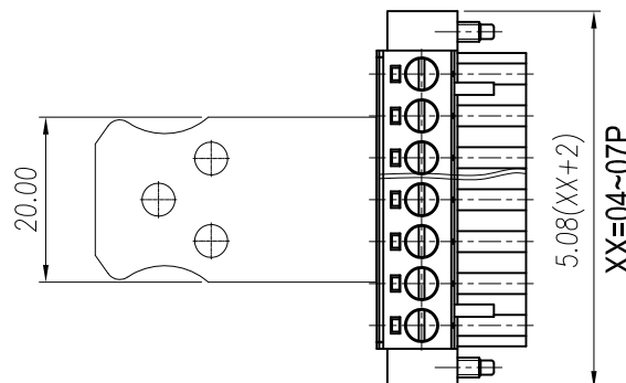
04~07P尺寸图
